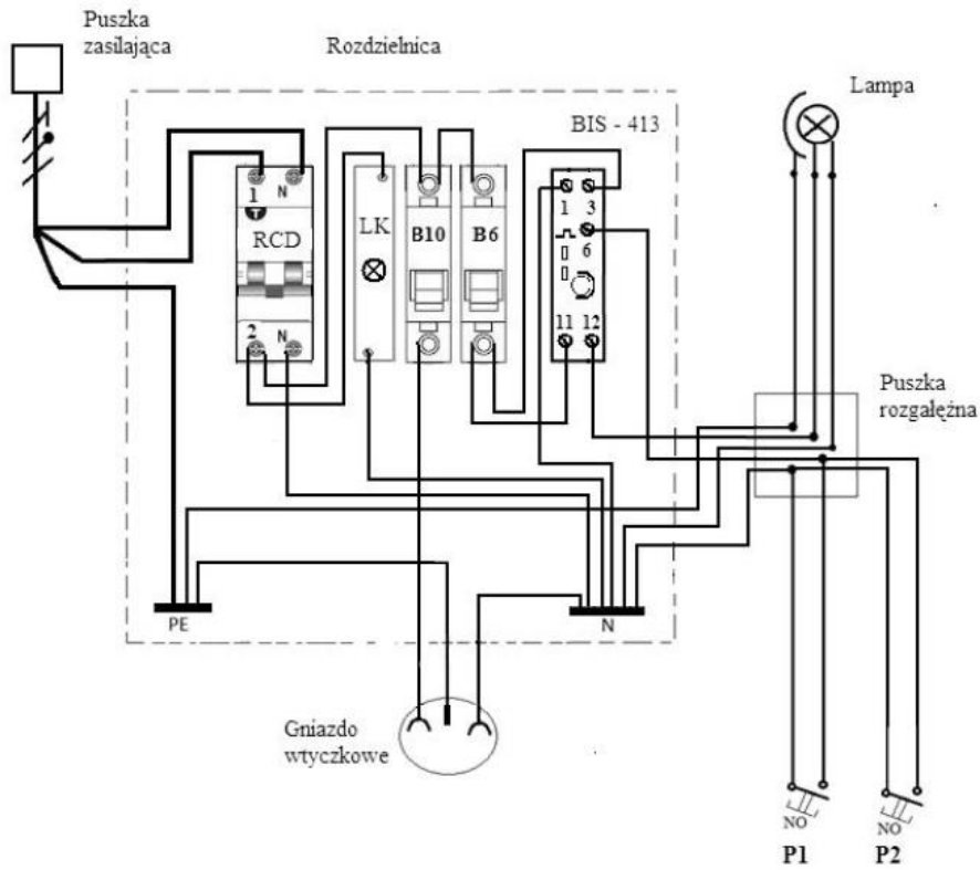
Rys.1. Schemat montażowy instalacji.
